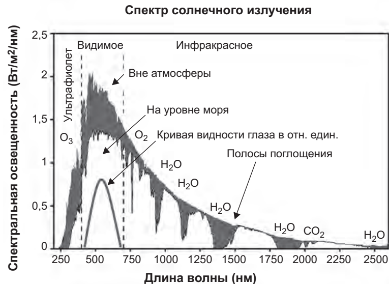
Рис. 1.5. Энергетический спектр солнечного излучения до его входа в атмосферу (серая заливка) и на уровне моря при отсутствии облачности (белая заливка); провалы на белой заливке — полосы его поглощения атмосферой Земли. Около каждой полосы поглощения указаны поглощающие газы [Ортенберг, Трифионов, 1990]. Серая кривая дневной чувствительности глаза с пиком на 555 нм дана в относительных единицах, не связанных с размерностью оси ординат
