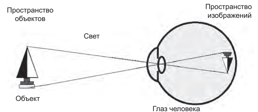
Рис. 1.3. Оптическое описание объекта; построение изображения в глазу человека
